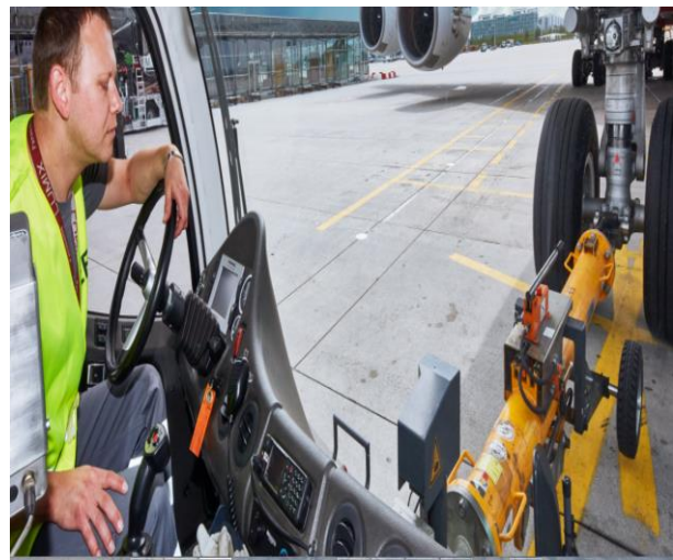
1. ábra: Merev vontatótengelyes repülőgép vontató
